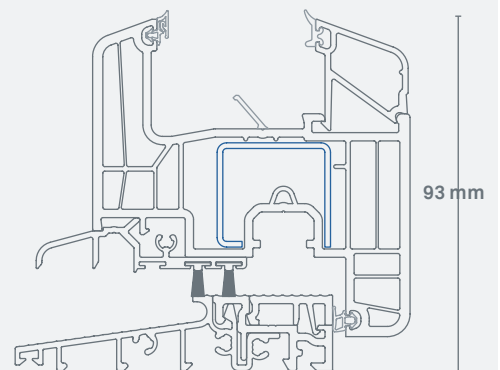
Nowość : Bezbarierowy próg do drzwi balkonowych Rys.: 1:2
